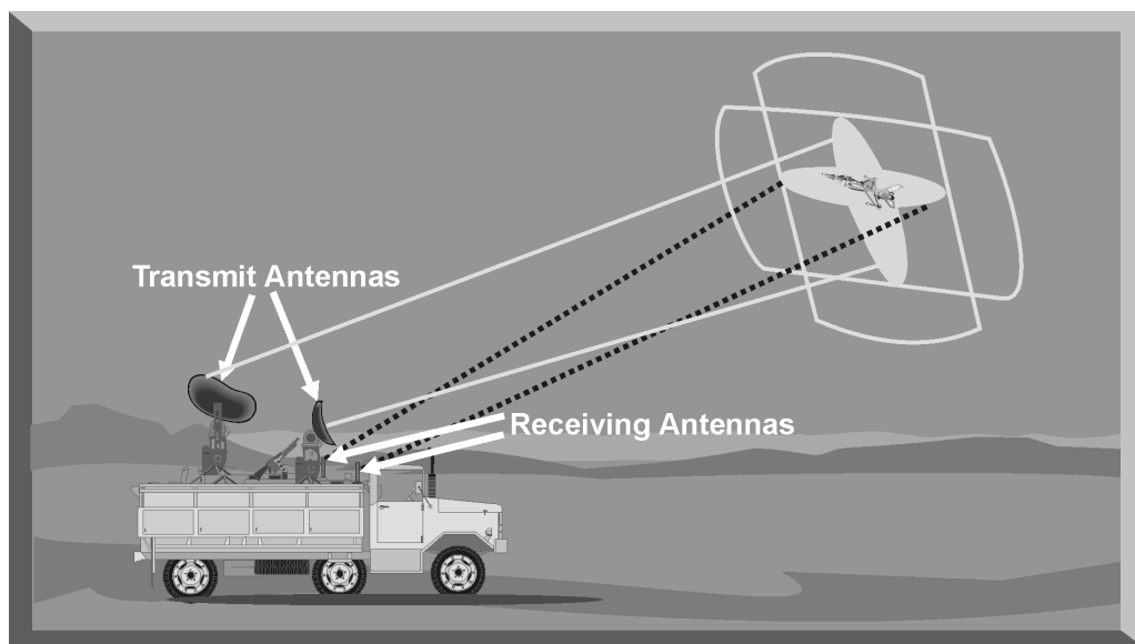
Figure 7-12. LORO Mode
